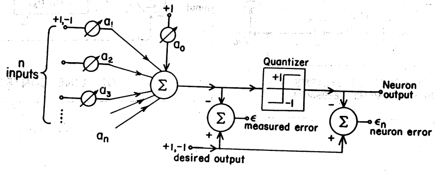
Fig. 12 ADALINE
